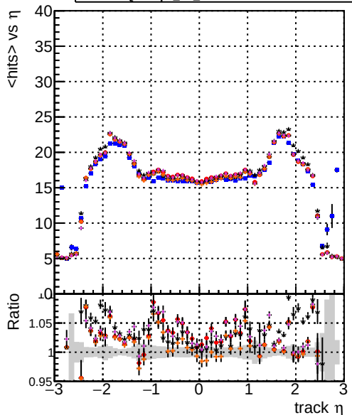
DOMstep3 TT CKF DOMstep3 TT default DOMstep3 TT ckrPixelLess DOMstep3 TT default1 DOMstep3 TT defaultNEWTOLDSAMPLE
