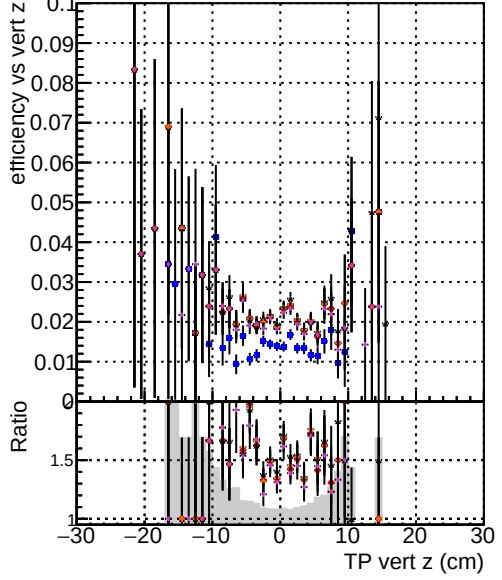
Efficiency vs. TP vert z (cm) DOMstep3 CKF DOMstep3 default DOMstep3 ckrPixelLess DOMstep3 default1 DOMstep3 defaultNEWTOLDSAMPLE
