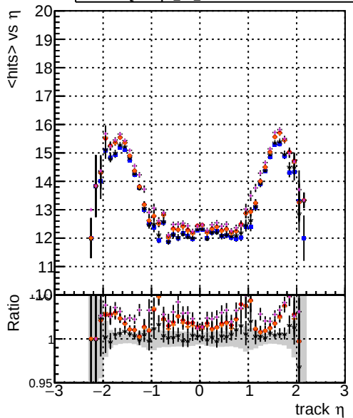
mean hit DOMstep3 CKF default DOMstep3 CKFPixelLess DOMstep3 default1 DOMstep3 defaultNEWTOLDSAMPLE
