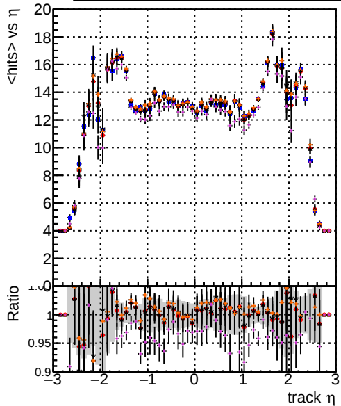
mean hits vs \eta DOMstep3 TT CKF DOMstep3 TT default DOMstep3 TT ckrPixelLess DOMstep3 TT default1 DOMstep3 TT defaultNEWTOLDSAMPLE
