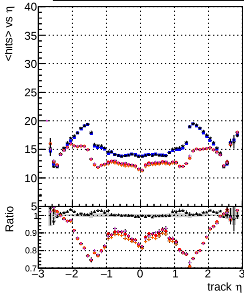
mean hits DOMstep3 TT CKF DOMstep3 TT default DOMstep3 TT ckPixelLess DOMstep3 TT default1 DOMstep3 TT default1NEWTOLDSAMPLE
