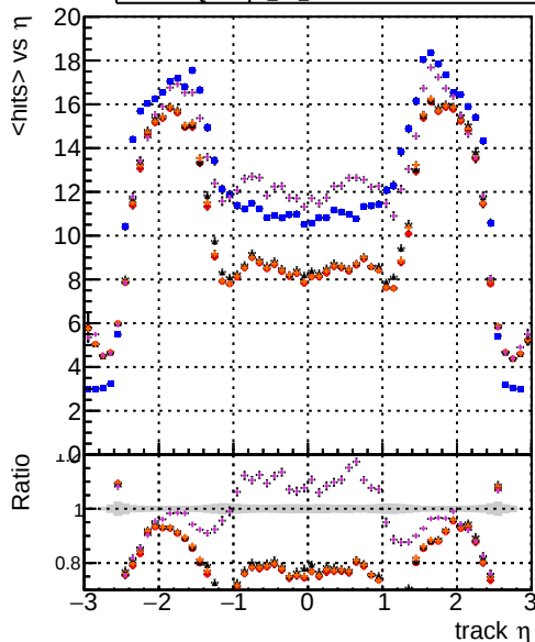
mean hits DOMstep3 TT CKF DOMstep3 TT default DOMstep3 TT ckPixelLess DOMstep3 TT default1 DOMstep3 TT defaultNEWTOLDSAMPLE
