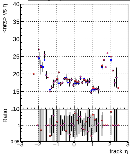
mean hit DOMstep3 TT CKF DOMstep3 TT default DOMstep3 TT ckPixelLess DOMstep3 TT default1 DOMstep3 TT default1NEWTOLDSAMPLE
