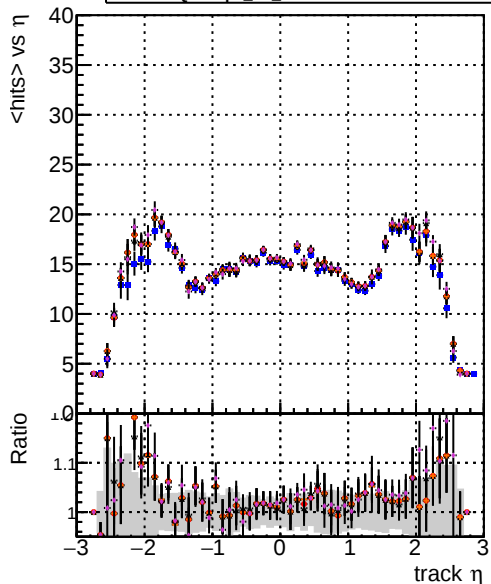
DOMstep3 TT CKF DOMstep3 TT default DOMstep3 TT CKPixelLess DOMstep3 TT default1 DOMstep3 TT defaultNEWTOLDSAMPLE mean hits
