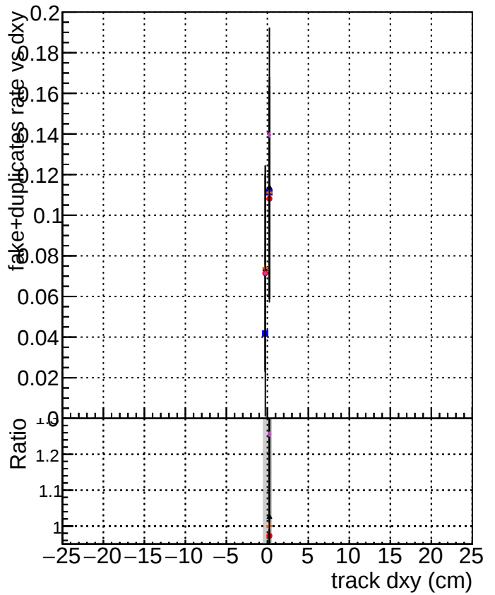
DQMstep3_TT_CKF DQMstep3_TT_default DQMstep3_TT_ckfPixelLess DQMstep3_TT_default1 DQMstep3_TT_defaultNEWTOLDSAMPLE
