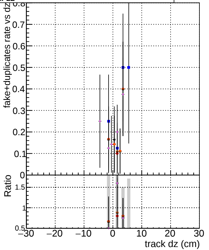
DQMstep3_TT_CKF DQMstep3_TT_default DQMstep3_TT_ckfPixelLess DQMstep3_TT_default1 DQMstep3_TT_defaultNEWTOLDSAMPLE
