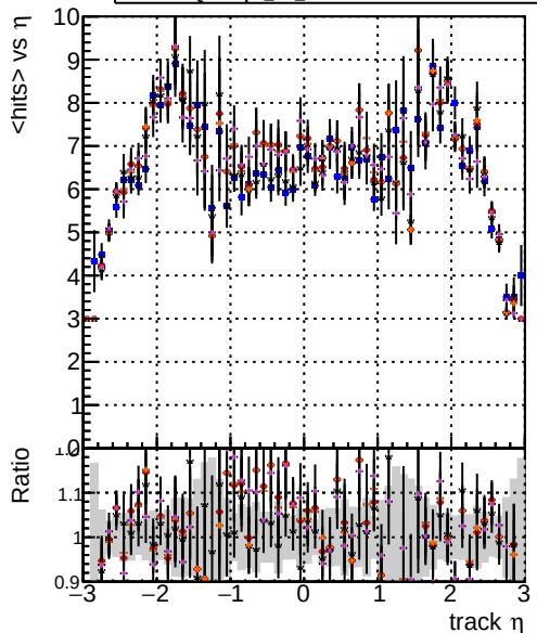
DOMstep3 TT CKF DOMstep3 TT default DOMstep3 TT ckfPixelLess DOMstep3 TT default1 DOMstep3 TT defaultNEWTOLDSAMPLE mean hit
