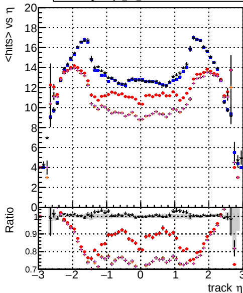
mean hits DOMstep3 CKF DOMstep3 ckPixelLess DOMstep3 default DOMstep3 default1 DOMstep3 defaultNEWTOLDSAMPLE
