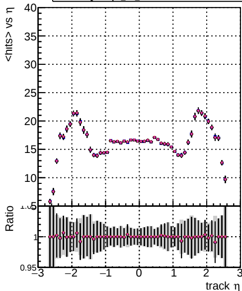
mean hits DOMstep3 TT CKF DOMstep3 TT default DOMstep3 TT ckfPixelLess DOMstep3 TT default1 DOMstep3 TT default1NEWTOLDSAMPLE
