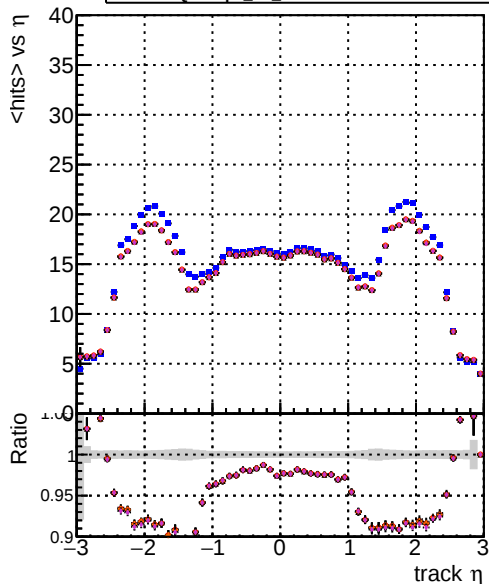
mean hit DOMstep3 TT CKF DOMstep3 TT default DOMstep3 TT CKPixelLess DOMstep3 TT default1 DOMstep3 TT defaultNEWTOLDSAMPLE
