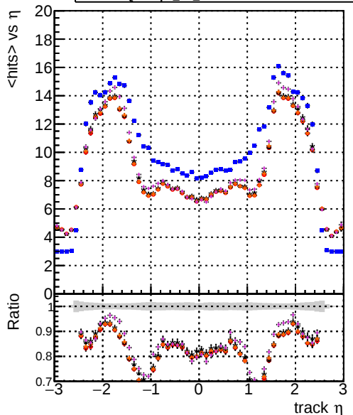
mean hit DOMstep3 TT CKF DOMstep3 TT default DOMstep3 TT ckfPixelLess DOMstep3 TT default1 DOMstep3 TT default1NEWTOLDSAMPLE
