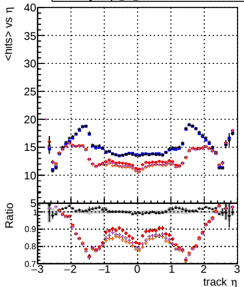
mean hits vs \eta DOMstep3 TT CKF DOMstep3 TT default DOMstep3 TT CKPixelLess DOMstep3 TT default1 DOMstep3 TT defaultNEWTOLDSAMPLE
