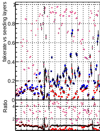
Fake rate vs. DOMstep3 DOMstep3+GKE DOMstep3+GKE+default-refr
