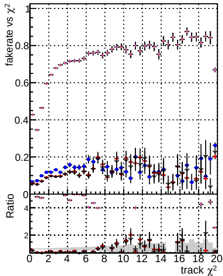
Fake rate vs. DOMstep3 DOMstep3+ GKE default-refr
