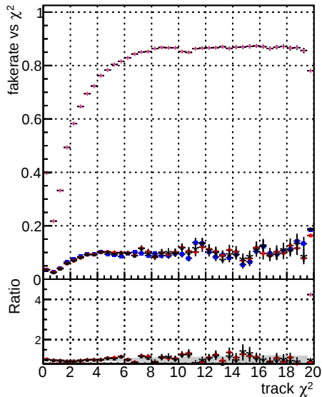
Fake rate vs. DOMstep3 DOMstep3+GKF DOMstep3+GKF+default-ref
