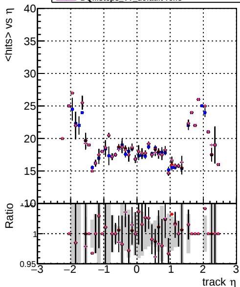
mean hit DOMstep3 CKF DOMstep3 default DOMstep3 CKPixelLess DOMstep3 default-ref4 DOMstep3 default-ref5
