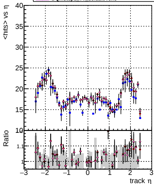
mean hits vs \eta DOMstep3 CKF DOMstep3 default DOMstep3 CKPixelLess DOMstep3 default-ref4 DOMstep3 default-ref5
