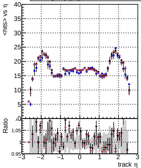
mean hit DOMstep3 CKF DOMstep3 CKFPixelLess DOMstep3 default-relf4 DOMstep3 default-relf5
