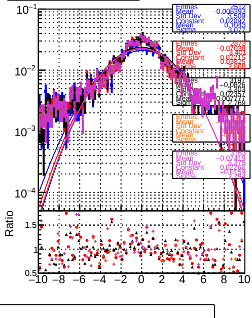
pull of \theta parameter
