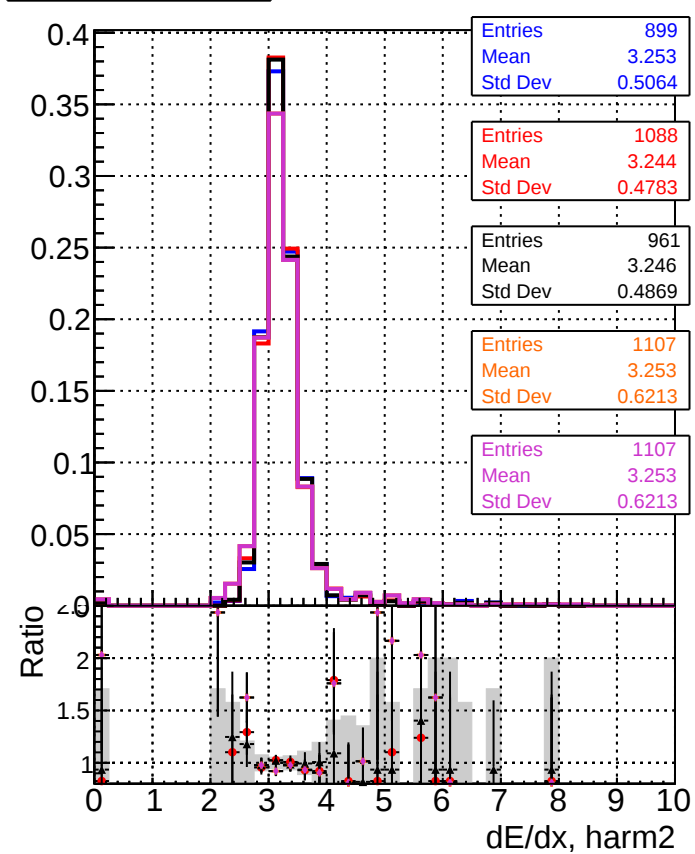
DOMstep3 TT CKF DOMstep3 TT default DOMstep3 TT ckfPixelLess DOMstep3 TT default-relf4 DOMstep3 TT default-relf5
