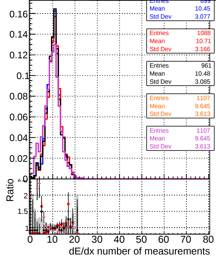
DOMstep3 TT CKF DOMstep3 TT default DOMstep3 TT ckfPixelLess DOMstep3 TT default-relf4 DOMstep3 TT default-relf5
