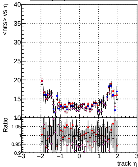
mean hit DOMstep3 CKF DOMstep3 ckrPixelLess DOMstep3 default-relf4 DOMstep3 default-relf5
