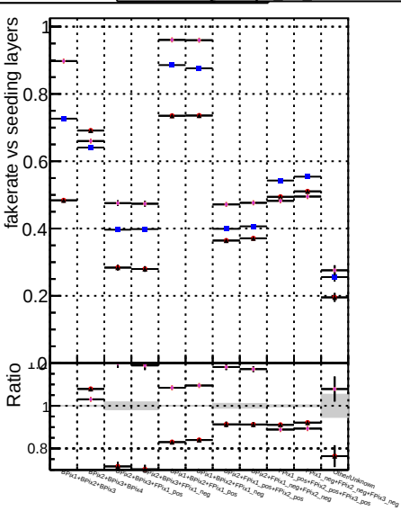
Fake rate vs. DOMstep3 DOMstep3+GKF DOMstep3+GKF+PileupLess
