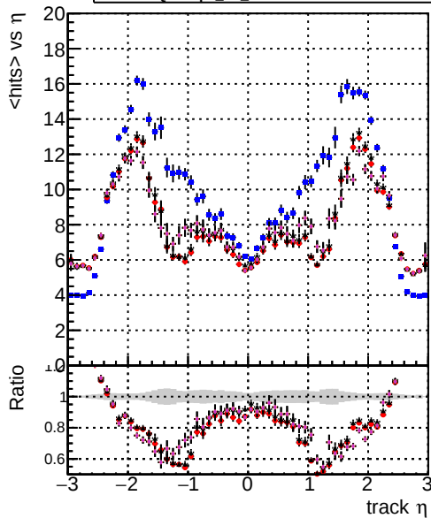
mean hits vs \eta DOMstep3 TT CKF DOMstep3 TT default DOMstep3 TT ckPixelLess DOMstep3 TT default-ref4 DOMstep3 TT default-ref5
