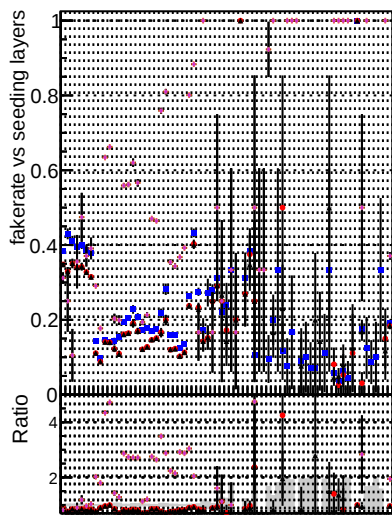
Fake rate vs. DOMstep3 DOMstep3+GKF DOMstep3+GKF+default+reco DOMstep3+GKF+default+reco+less
