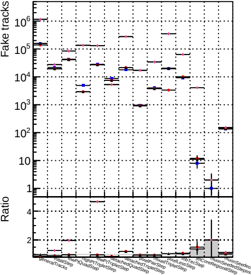
Number Parameter Value 1 DOMstep3 TT CKFixeILess 2 DOMstep3 TT default-relf4 3 DOMstep3 TT defaultNEWTOLDSAMPLE-relf4
