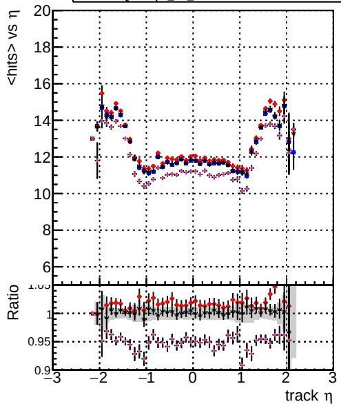
DOMstep3 CKF DOMstep3 default DOMstep3 ckPixelLess DOMstep3 default-relf4 DOMstep3 default-NEWTOLDSAMPLE-relf4 mean hits
