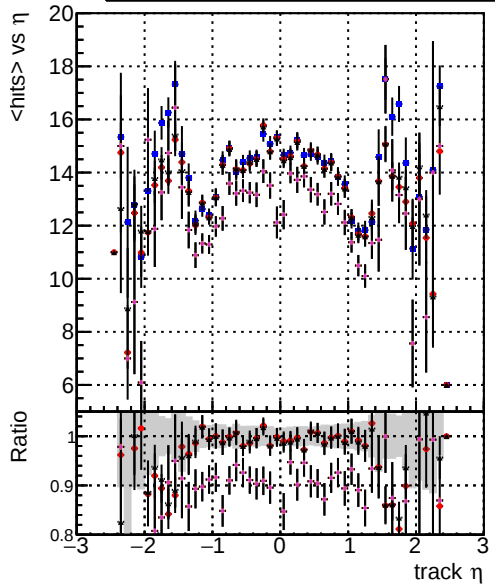
mean hits DOMstep3 TT CKF DOMstep3 TT default DOMstep3 TT ckfPixelLess DOMstep3 TT default-relf4 DOMstep3 TT defaultNEWTOLDSAMPLE-relf4
