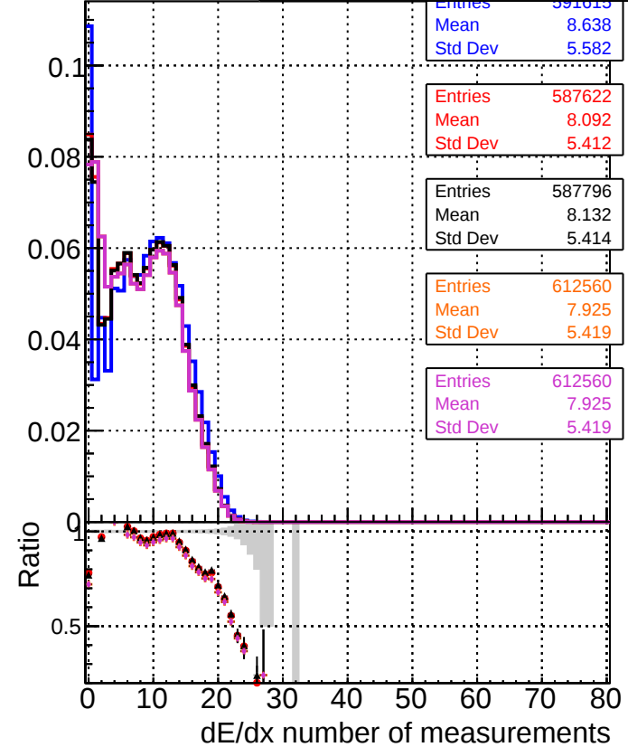
DOMstep3 TT CKF DOMstep3 TT default DOMstep3 TT ckfPixelLess DOMstep3 TT default-rlf4 DOMstep3 TT defaultNEWTOLDSAMPLE-rlf4
