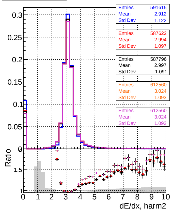
DOMstep3 TT CKF DOMstep3 TT default DOMstep3 TT ckfPixelLess DOMstep3 TT default-rlf4 DOMstep3 TT defaultNEWTOLDSAMPLE-rlf4
