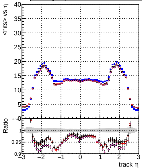
mean hit DOMstep3 TT CKF DOMstep3 TT default DOMstep3 TT ckPixelLess DOMstep3 TT default-relf4 DOMstep3 TT defaultNEWTOLDSAMPLE-relf4
