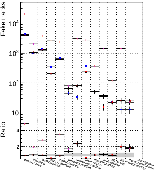
Number Symbol Parameter ▲ DOMstep3 TT ckrPixelLess ● DOMstep3 TT default-relf4 ○ DOMstep3 TT defaultNEWTOLDSAMPLE-relf4
