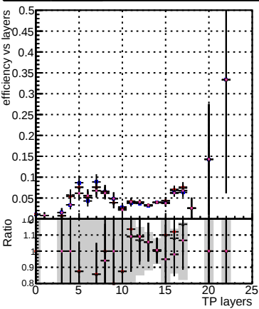
Efficiency vs hit Legend: DOMstep3 TT_CKF DOMstep3 TT_default DOMstep3 TT_ckfPixelLess DOMstep3 TT_default-relf4 DOMstep3 TT_defaultNEWTOLDSAMPLE-relf4
