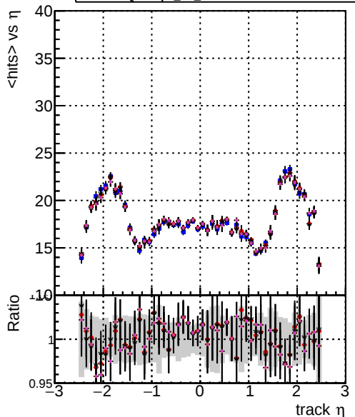
DQMstep3 TT CKF DQMstep3 TT default DQMstep3 TT ckfPixelLess DQMstep3 TT default-relf4 DQMstep3 TT defaultNEWTOLDSAMPLE-relf4 mean hit
