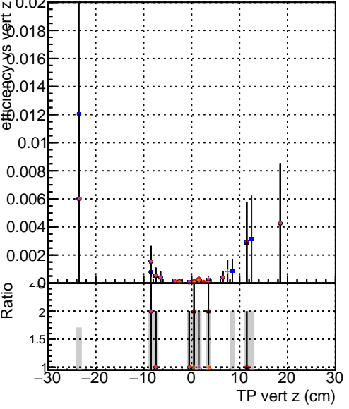
Efficiency vs vertpos — DQMstep3 — CKF ● DQMstep3 — default ● DQMstep3 — CKF+PixelLess ● DQMstep3 — default+relf3 ● DQMstep3 — default+NEWTOLDSAMPLE+relf3
