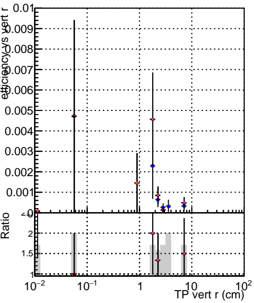
Efficiency vs vertpos — DQMstep3 — CKF ● DQMstep3 — default ● DQMstep3 — CKF+PixelLess ● DQMstep3 — default+relf3 ● DQMstep3 — default+NEWTOLDSAMPLE+relf3
