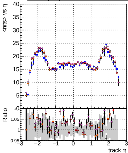
mean hits vs \eta DOMstep3 TT CKF DOMstep3 TT default DOMstep3 TT ckPixelLess DOMstep3 TT default-refl3 DOMstep3 TT defaultNEWTOLDSAMPLE-refl3
