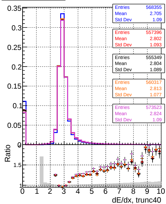
— DQMstep3 TT CKF — DQMstep3 TT default — DQMstep3 TT ckfPixelLess — DQMstep3 TT default-rlf3 — DQMstep3 TT defaultNEWTOLDSAMPLE-rlf3
