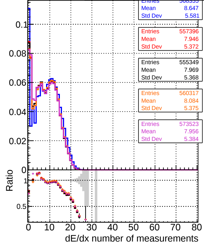
— DQMstep3 TT CKF — DQMstep3 TT default — DQMstep3 TT ckfPixelLess — DQMstep3 TT default-rlf3 — DQMstep3 TT defaultNEWTOLDSAMPLE-rlf3
