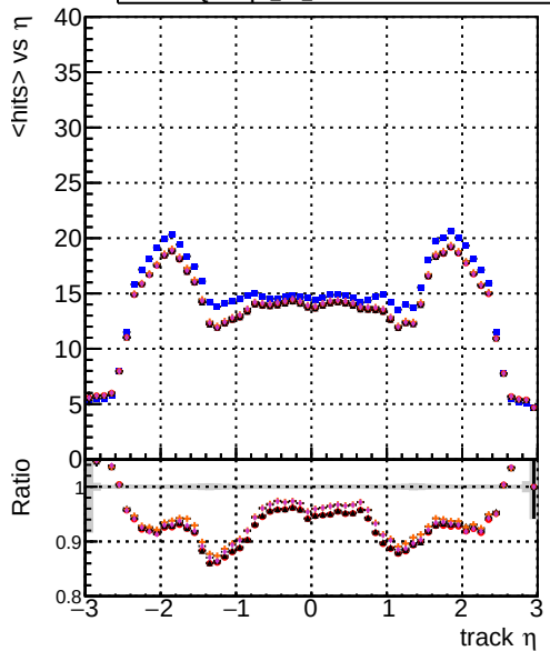
mean hits DOMstep3 TT CKF DOMstep3 TT default DOMstep3 TT ckPixelLess DOMstep3 TT default-relf3 DOMstep3 TT defaultNEWTOLDSAMPLE-relf3
