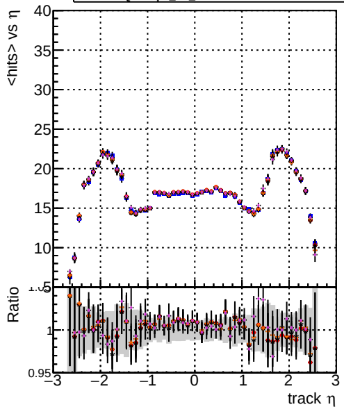
mean hits DOMstep3 TT CKF DOMstep3 TT default DOMstep3 TT CKPixelLess DOMstep3 TT default-rlf3 DOMstep3 TT defaultNEWTOLDSAMPLE-rlf3
