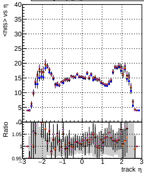
DOMstep3 TT CKF DOMstep3 TT default DOMstep3 TT ckPixelLess DOMstep3 TT default-relf3 DOMstep3 TT defaultNEWTOLDSAMPLE-relf3 mean hits
