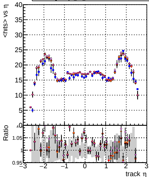
mean hits DOMstep3 TT CKF DOMstep3 TT default DOMstep3 TT ckPixelLess DOMstep3 TT default-refl3 DOMstep3 TT defaultNEWTOLDSAMPLE-refl3
