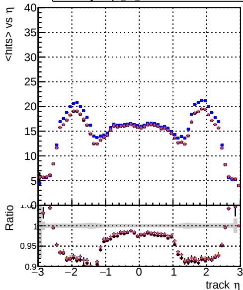
mean hits DOMstep3 TT CKF DOMstep3 TT default DOMstep3 TT CKPixelLess DOMstep3 TT default-relf3 DOMstep3 TT defaultNEWTOLDSAMPLE-relf3
