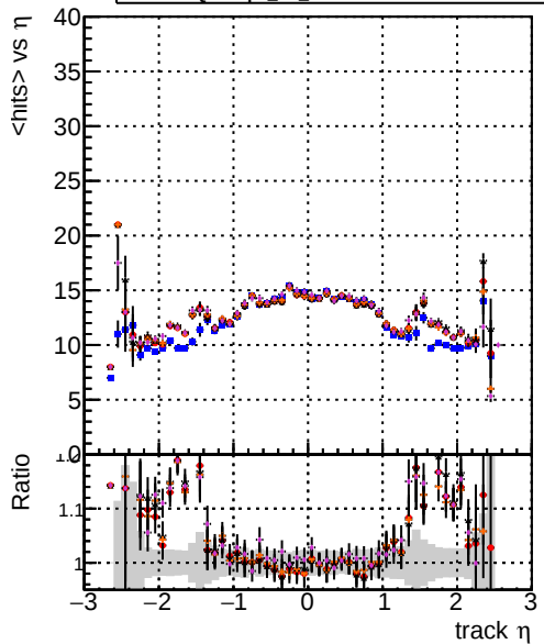
mean hits vs \eta DOMstep3 TT CKF DOMstep3 TT default DOMstep3 TT ckPixelLess DOMstep3 TT default-rlf3 DOMstep3 TT defaultNEWTOLDSAMPLE-rlf3
