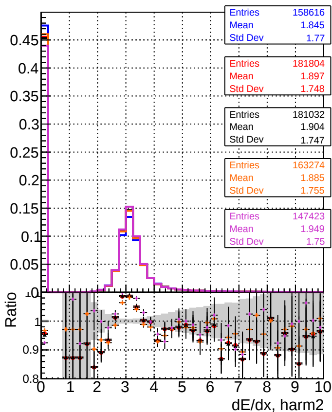
dE/dx estimator 1
