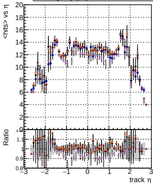
mean hits DOMstep3 TT CKF DOMstep3 TT default DOMstep3 TT ckfPixelLess DOMstep3 TT default-refl2 DOMstep3 TT defaultNEWTOLDSAMPLE-refl2
