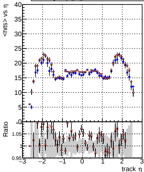
DOMstep3 TT CKF DOMstep3 TT default DOMstep3 TT ckPixelLess DOMstep3 TT default-ref12 DOMstep3 TT default-NEWTOLDSAMPLE-ref12 mean hits
