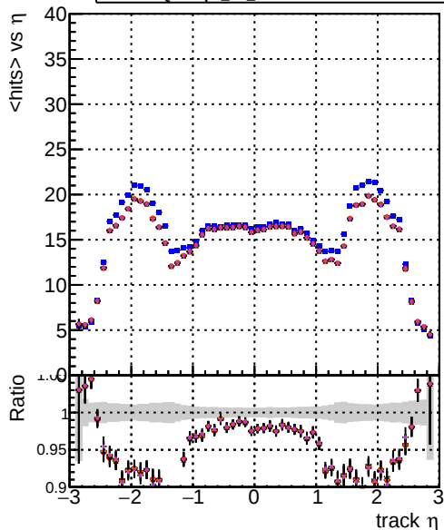
mean hits DOMstep3 CKF DOMstep3 default DOMstep3 CKPixelLess DOMstep3 default-refl2 DOMstep3 defaultNEWTOLDSAMPLE-refl2
