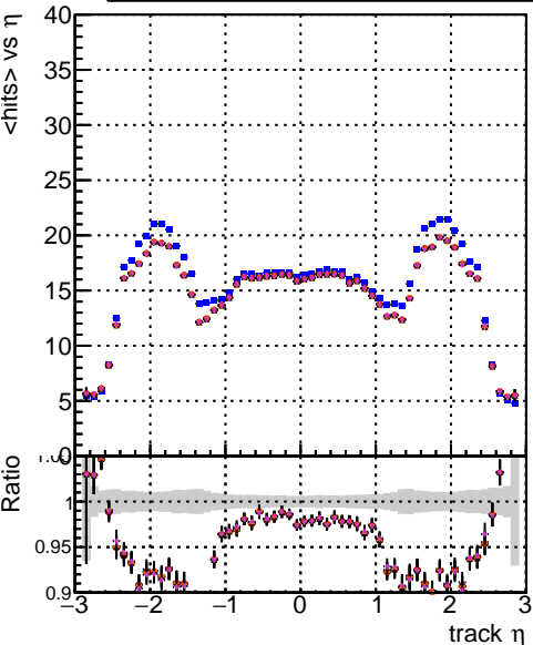
mean hit █ DQMstep3 CKF █ DQMstep3 default █ DQMstep3 ckfFixLess █ DQMstep3 default-relf2 █ DQMstep3 default-NEWTOLDSAMPLE-relf2
