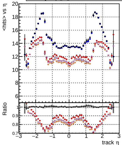
mean hits DOMstep3 CKF DOMstep3 default DOMstep3 ckPixelLess DOMstep3 default-refl2 DOMstep3 defaultNEWTOLDSAMPLE-refl2
